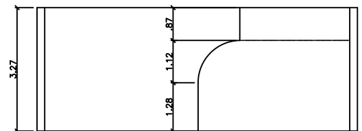
④ CORTE ESCADA B
