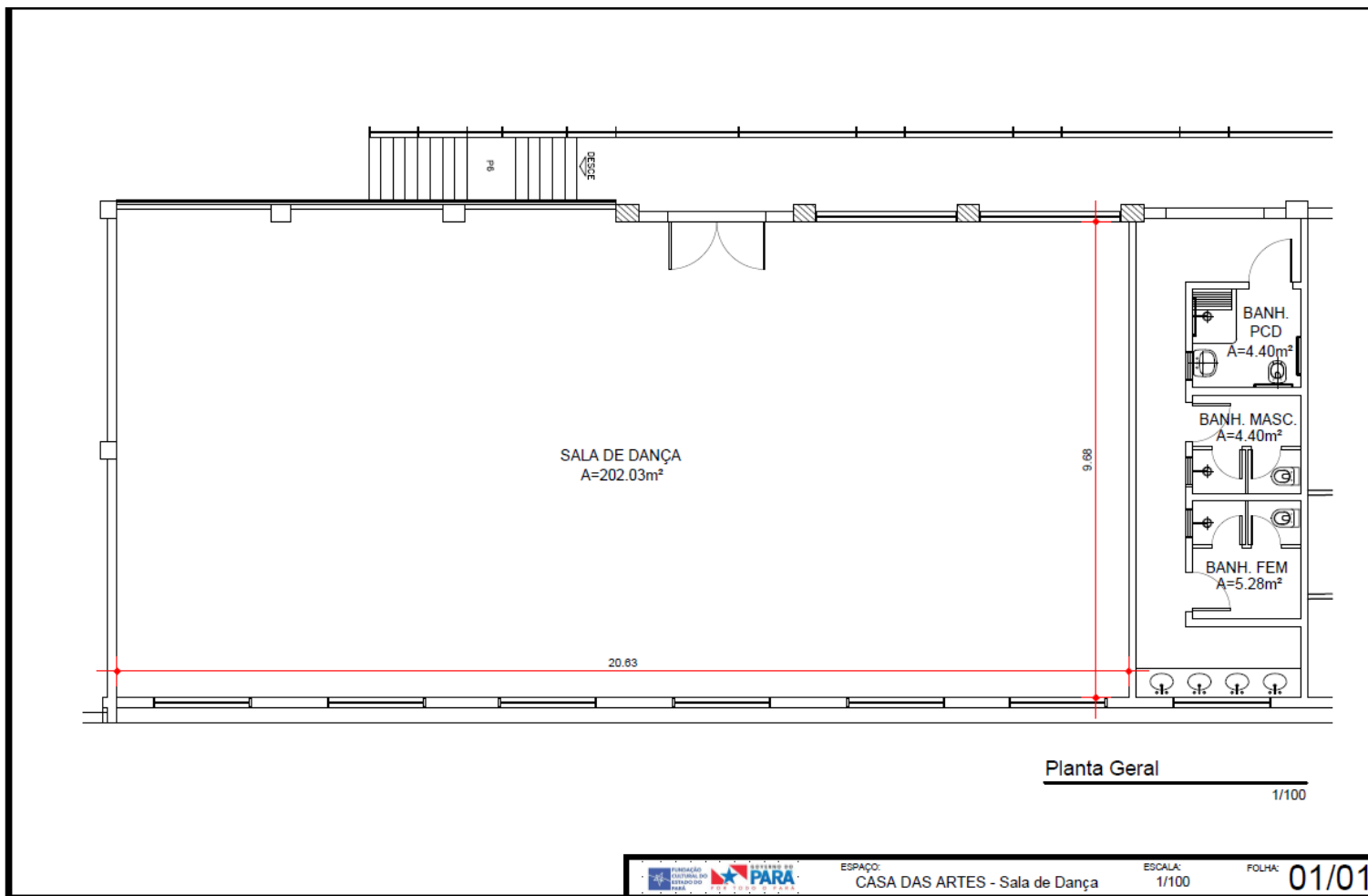
ANEXO 11 - PLANTA DA SALA DE DANÇA
